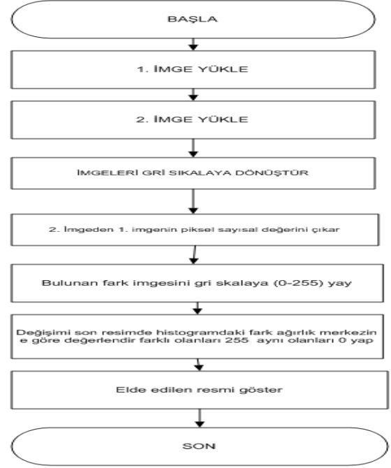
Şekil.12 İşleyişe ait algoritma
